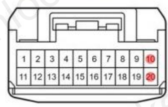
MULTIPLEX NETWORK DOOR ECU
